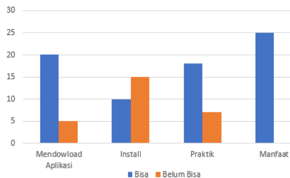
Gambar 5. Hasil Pelatihan
